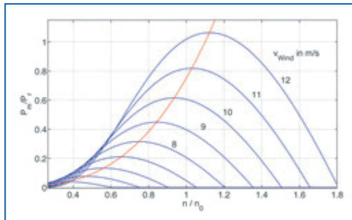
Bild 13 Die Kennlinie der mechanischen Leistung demonstriert das Verhältnis der mechanischen Leistung (Pm) zur Bemessungsleistung (Pr) in Abhängigkeit des Quotienten Drehzahl (n) zur Bemessungsdrehzahl (nr), bei entsprechender Windgeschwindigkeit (VWind) in Meter pro Sekunde pro Windrad [p(er) u(nit)]. Quelle: Institut für Energieversorgung und Hochspannungstechnik, Fachgebiet Elektronische Energieversorgung, Leibniz Universität Hannover
