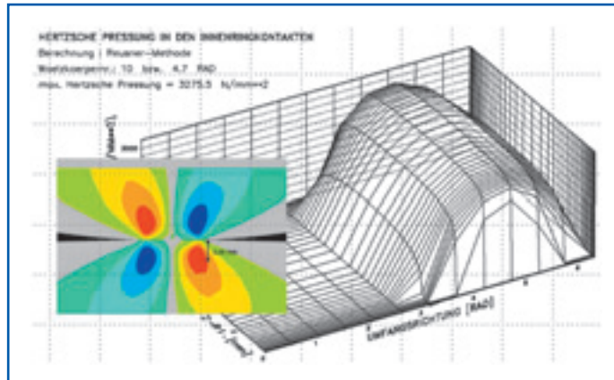
Bild 9 Hertzsche Pressung (größte Spannung, die in der Mitte der Berührungsfläche zweier elastischer Körper besteht) im Wälzkontakt ( D = \text{Dalton} , RAD = \text{Radiant} , N = \text{Newton} ) Quelle: Institut für Maschinenelemente, Konstruktionstechnik und Tribologie, Leibniz Universität Hannover
