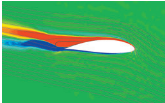
Bild 12 Turbulenz bei der Strömungsablösung an der Hinterkante eines Profils Quelle: Institut für Turbomaschinen und Fluid-Dynamik, Leibniz Universität Hannover
