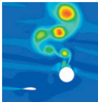
Bild 11 Wirbelschlepe bei der Turm-Blatt Interaktion: Gegenläufige Wirbel werden als Wirbelschlepe bezeichnet. Die Wirbelschlepe entsteht am umströmten Turmquerschnitt und wird durch das Zusammenspiel von Turm und Rotorblatt beeinflusst. Quelle: Institut für Turbomaschinen und Fluid-Dynamik, Leibniz Universität Hannover
