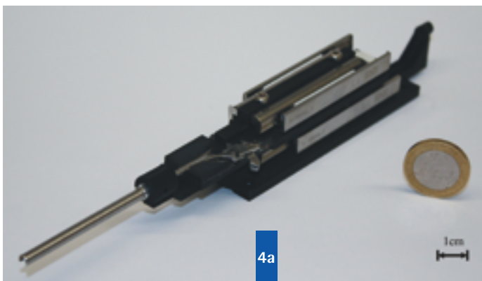
Abbildung 4 Automatisiertes Insertionstool für Cochlea-Implantate (oben)
