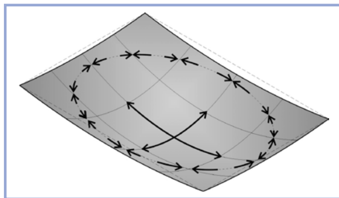
Abbildung 4 Mögliches Tragverhalten einer Decke im Brandfall (Membranwirkung)
