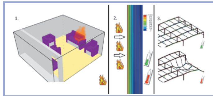
Abbildung 2 Teile einer vollständigen Trag- simulation im Brandfall – 1.) Brandsimulation; 2.) Tempe- raturesimulation in einer Beton- wand; 3.) Tragwerkssimulation mit kalten und heißen Bauteilen
