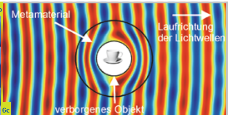
Abbildung 6 Dreidimensionales Laserschreiben durch Zwei-Photonen-Polymerisation (a) erlaubt die Herstellung von Mikroringen aus Polymer (b). Das Material kann selektiv mit einer Metallschicht überzogen werden. Die daraus entstehenden optischen Eigenschaften erlauben es, Lichtwellen um ein Objekt herumzuleiten, wie in einer Computersimulation dargestellt ist. Das Objekt im Zentrum erscheint für einen Beobachter als unsichtbar.
